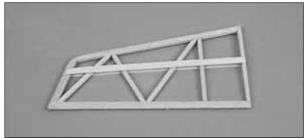
1/16" x 1/4" Stab Spars
