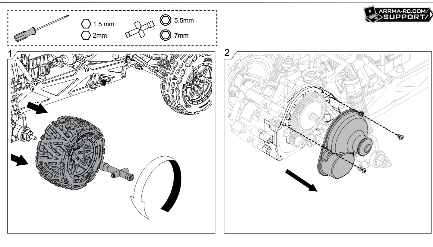
Motor Removal Ausbau des Motors Dépose du moteur Desmontaje del Motor モーターの取り外し 差速器移除和替换
